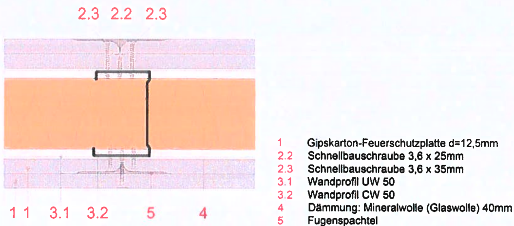
Abbildung 1 Horizontalschnitt – Stoßbereich der Gipskarton-Feuerschutzplatten (2lagige Ausführung) an einem mittleren Wandprofil
